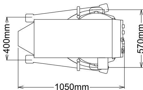
Felülnézet
