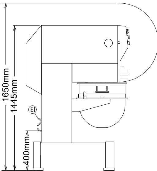
Oldalnézet
